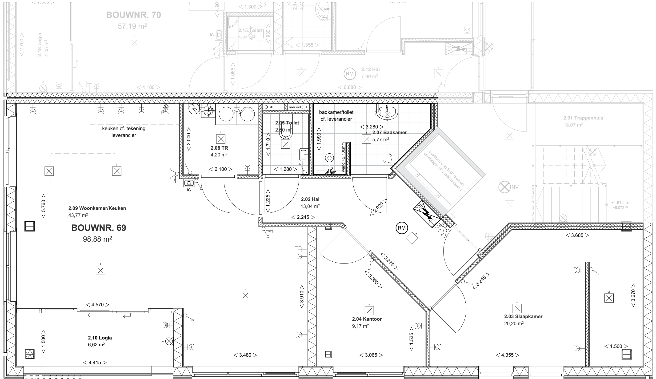
PLATTEGROND - 1:50
