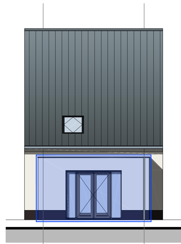
achtergevel 1:100 optie uitbouw 1.2m / 1.8m
