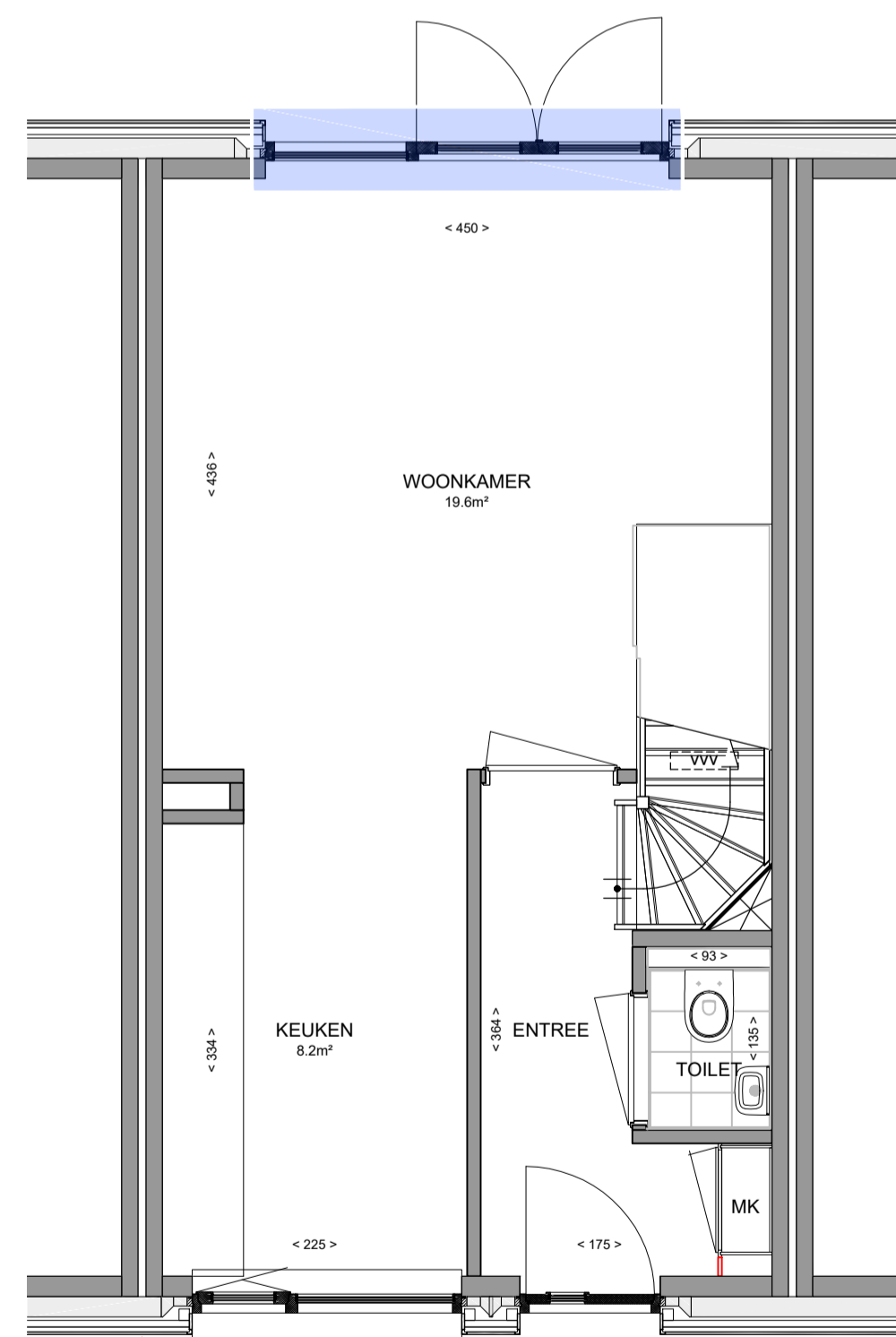
begane grond 1:50 optie openslaande deuren
