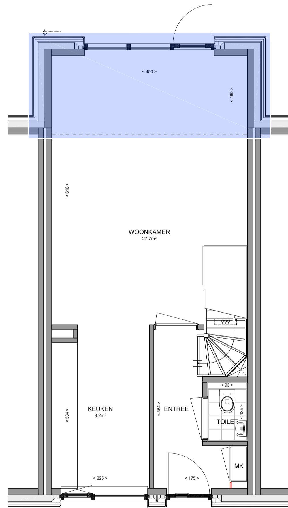
begane grond 1:50 optie uitbouw 1.8m
