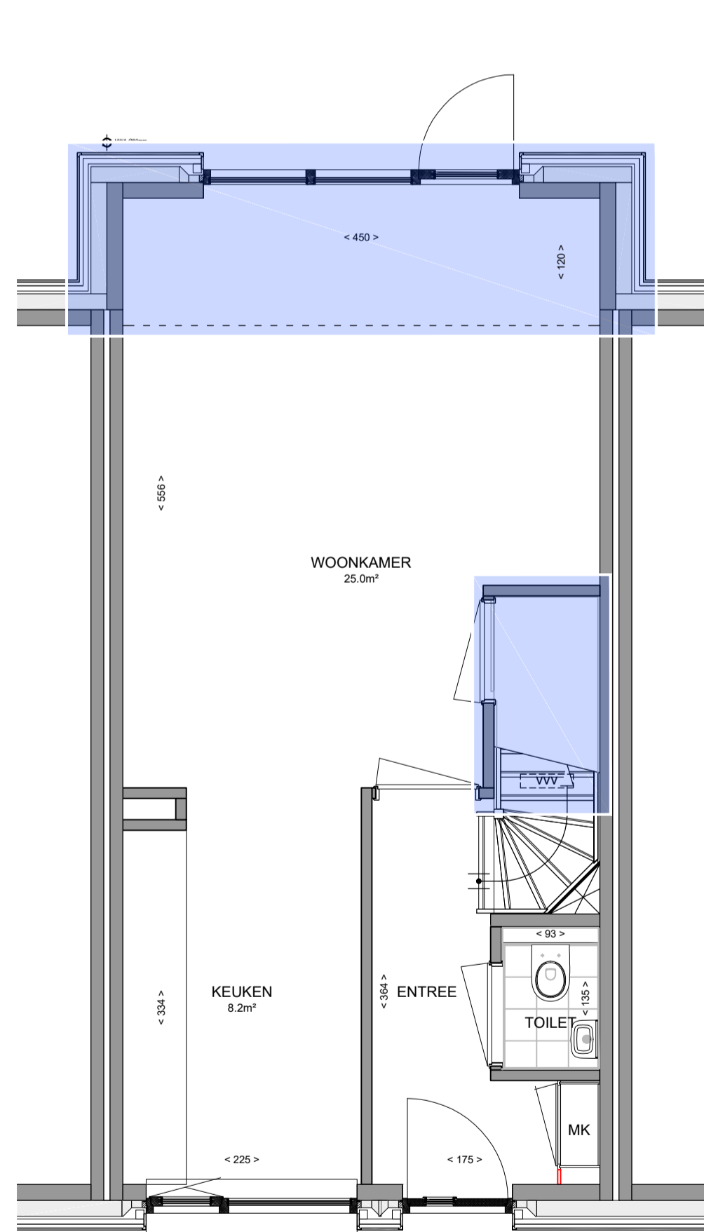
begane grond 1:50 optie uitbouw 1.2m optie trapkast
