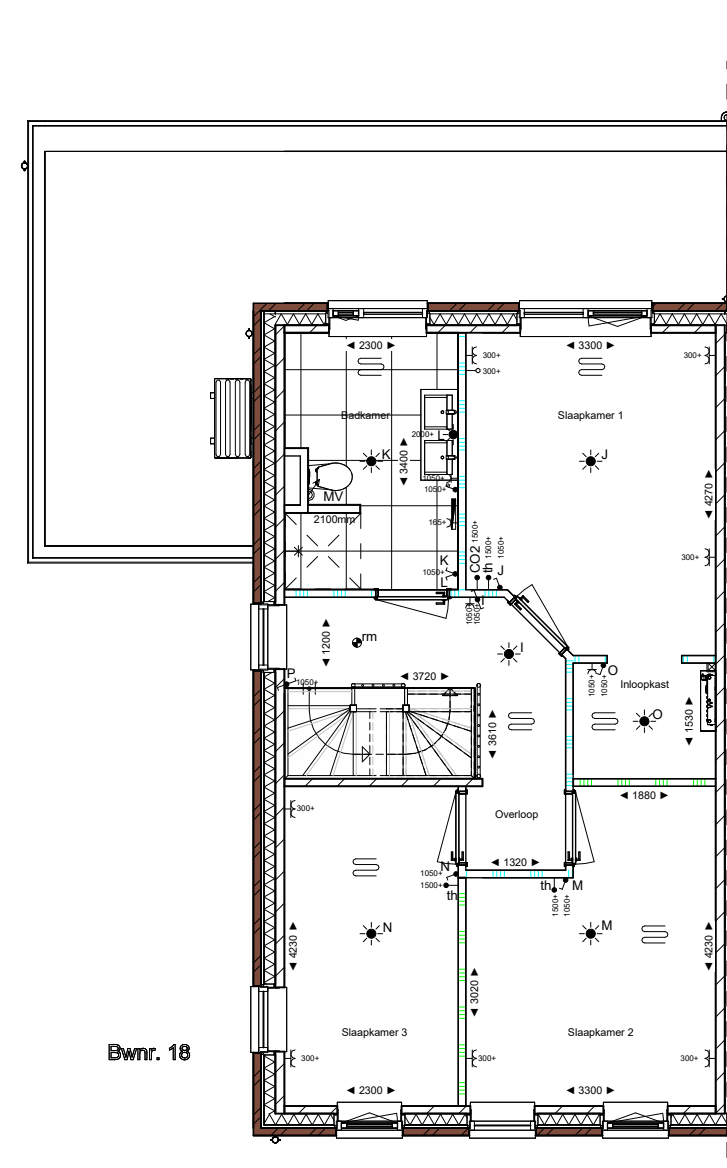
eerste verdieping
