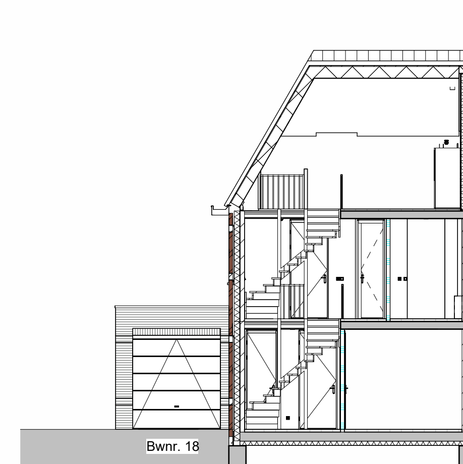
Doorsnede A_Bwnr. 18
