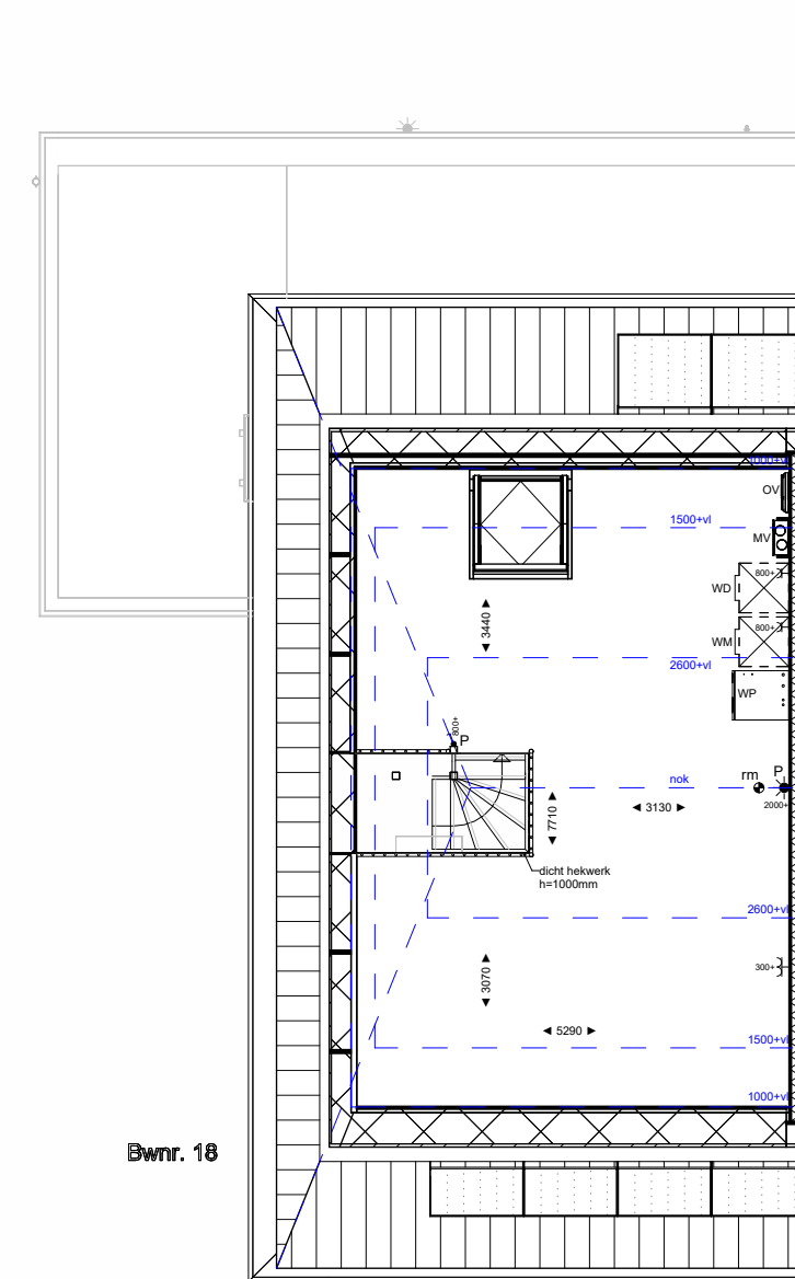
tweede verdieping
