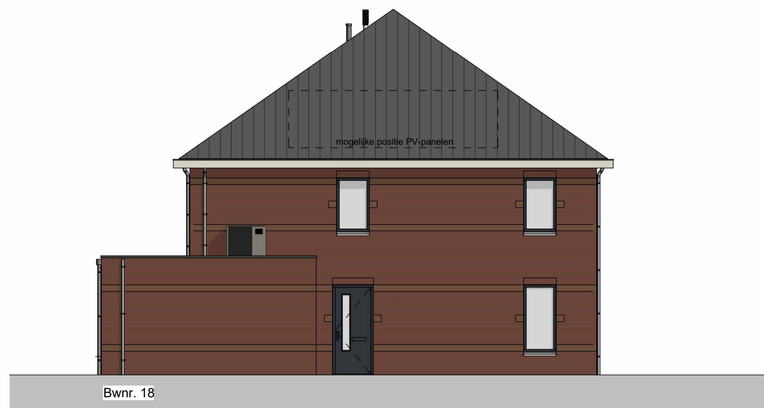
linkergevel
