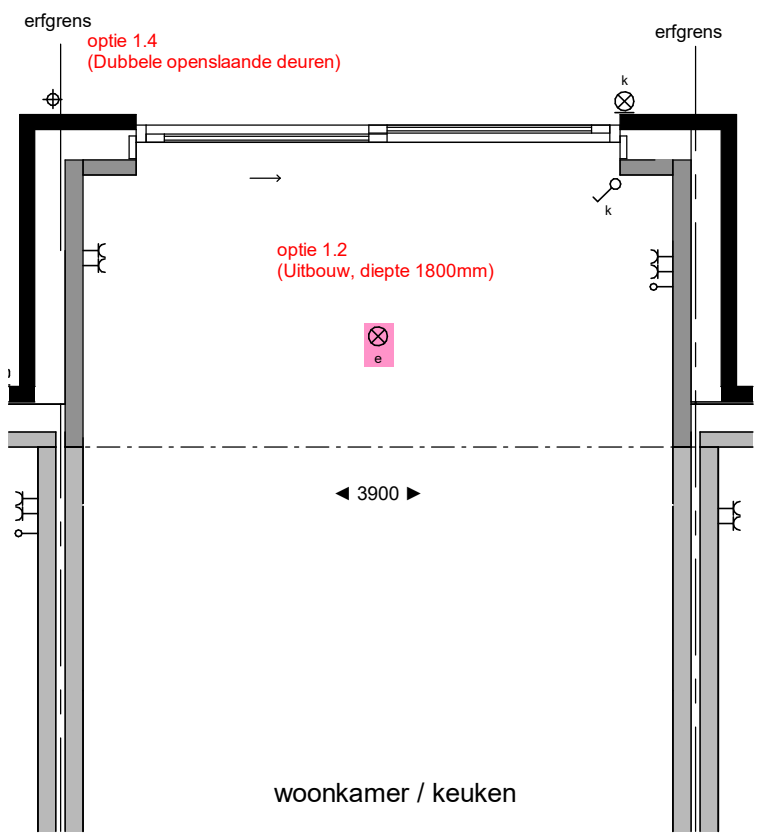
begane grond
