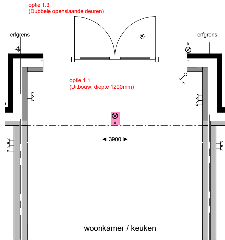
begane grond
