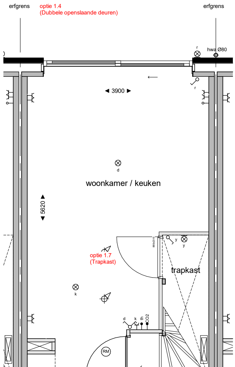
begane grond
